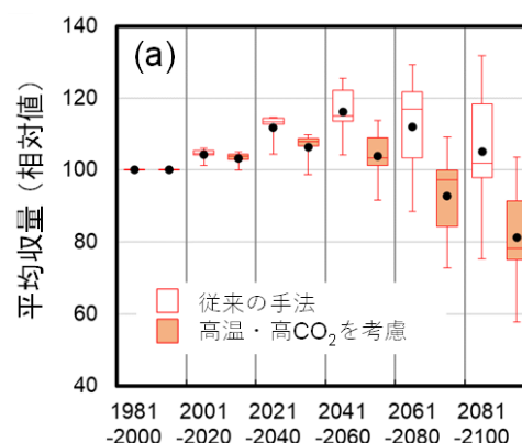
図. 高温・高 CO 2 の複合影響が考慮された水稻収量の 20 年毎の推移（全国平均）
